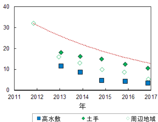
【図 2】場所ごとの空間線量率の時間変化 (赤破線は 2011 年 11 月 5 日の周辺地域の空間線量率からの自然減衰による減少分を示しています)
