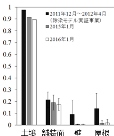
【図 3】土壌、舗装面、壁、屋根におけるセシウムの相対存在量
