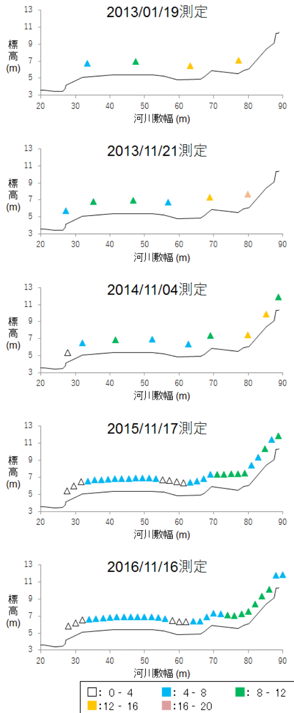
【図 1】 河川敷内の空間線量率分布と時間変化
