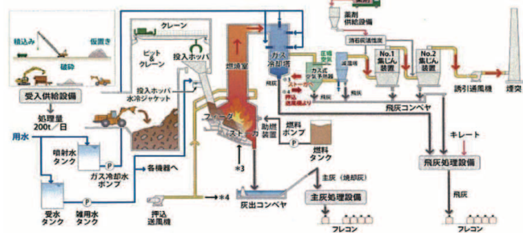
施設内設備フロー(図3)
